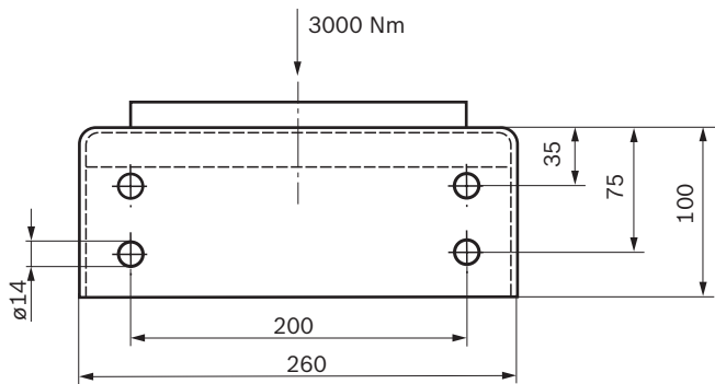
Konsole (Materialnummer: 1531334008)
