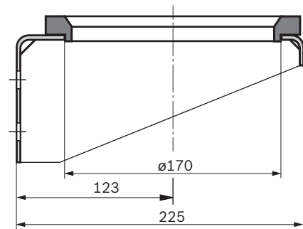
Gummistützring (Materialnummer 1530221042)
